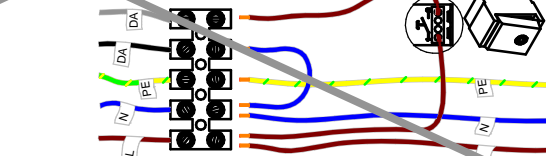
Cablaggio per gestione con pulsante "NA" - Wiring for operation with button "NA" - De cableado para la operación con el botón de "NA" - Câblage pour un fonctionnement avec le bouton "NA" - Verdrahtung für den Betrieb mit Button "NA"
