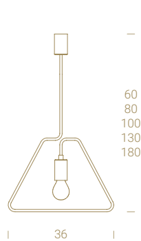
Sospensione · Suspension
